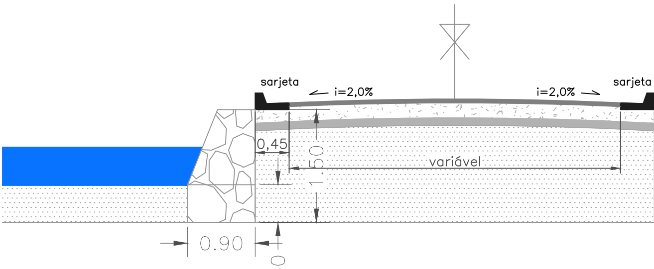
DETALHE DO MURO DE PEDRA ARGAMASSADA (meio fio c/ sarjeta) Esc.: 1/50
