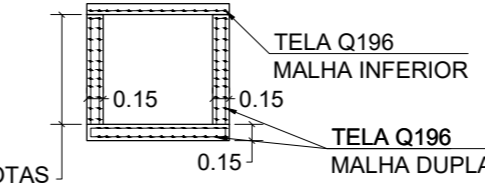
SEÇÃO TRANSVERSAL CORTE CC = CORTE DD
