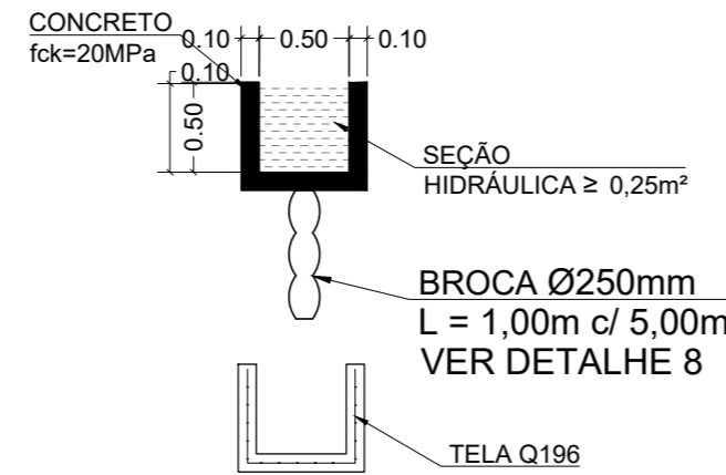
SEÇÃO TRANSVERSAL
