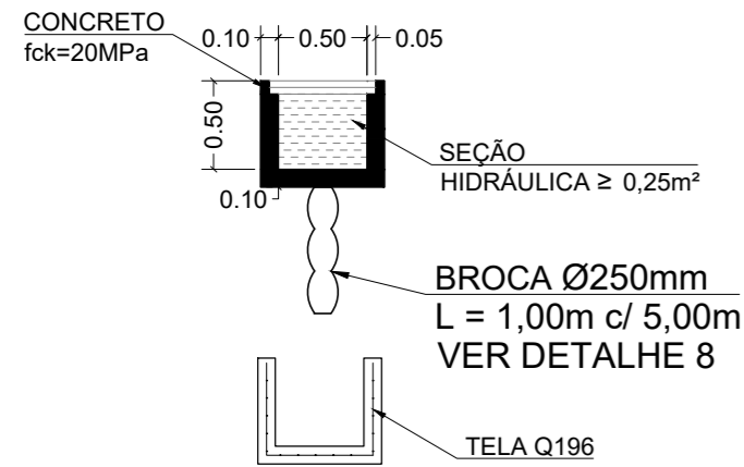
SEÇÃO TRANSVERSAL
