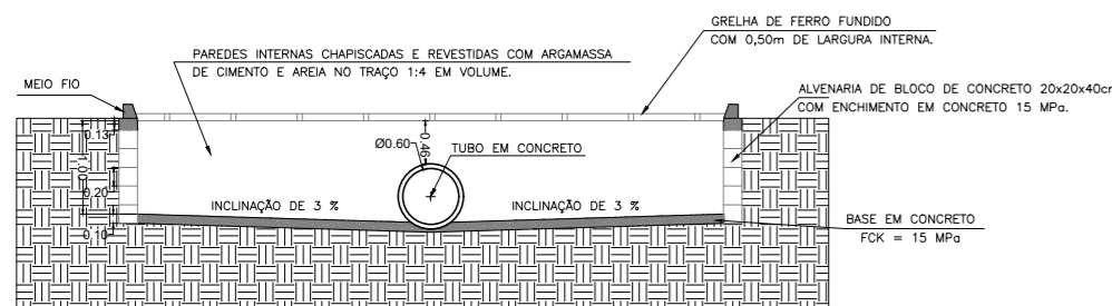
CORTE AA
