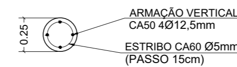
SEÇÃO TRANSVERSAL CORTE FF
