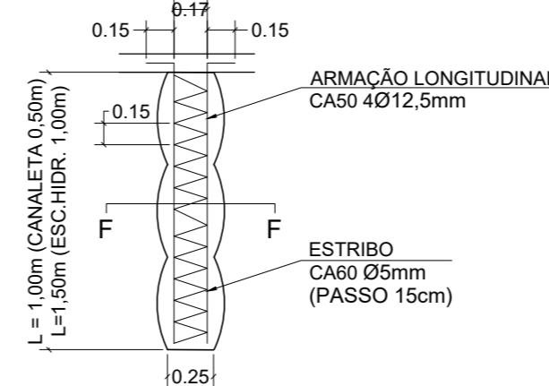
SEÇÃO LONGITUDINAL
