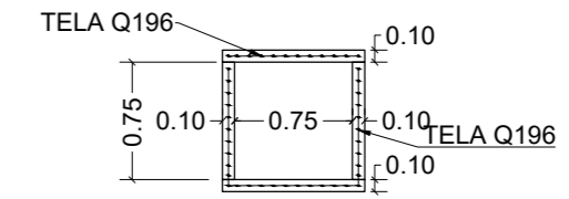
SEÇÃO TRANSVERSAL CORTE CC = CORTE DD
